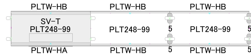
高架駅部分の「高架プレート」「側壁」「橋脚」の設置図
